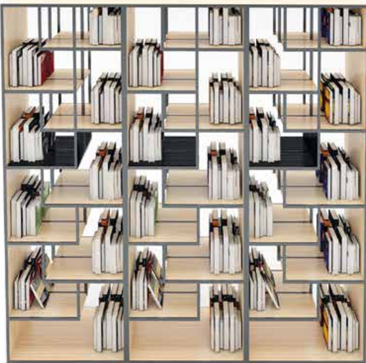
KTP - 02 - ÇİFT TARAFLI METAL KİTAPLIK L207 - W60 - H190
